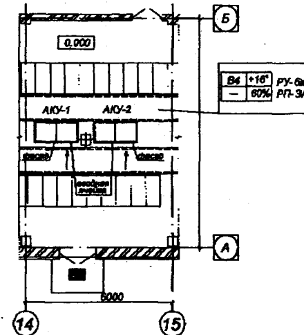
План расстановки конденсаторных установок
